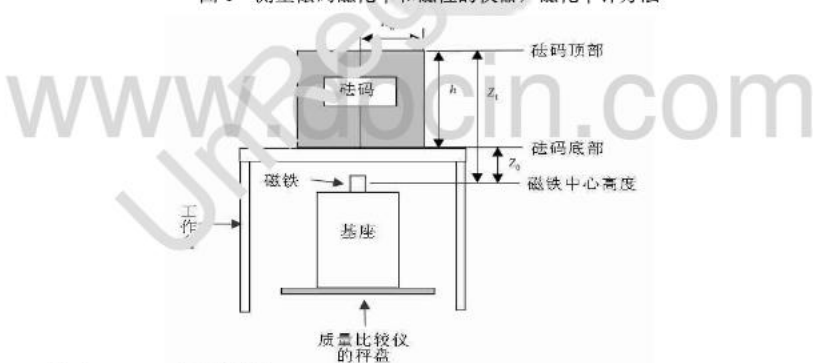
图 1 测量砝码磁化率和磁性的仪器, 磁化率计方法
